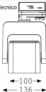
Disegno Tecnico
