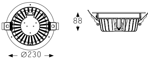
Disegno Tecnico
