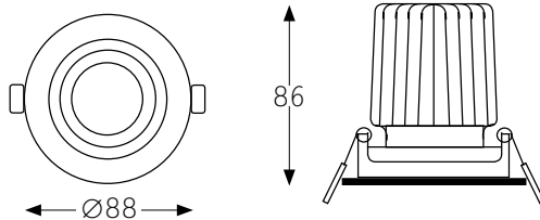
Disegno Tecnico
