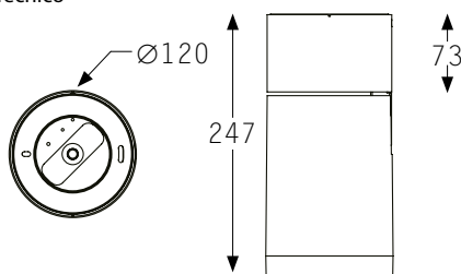
Disegno Tecnico
